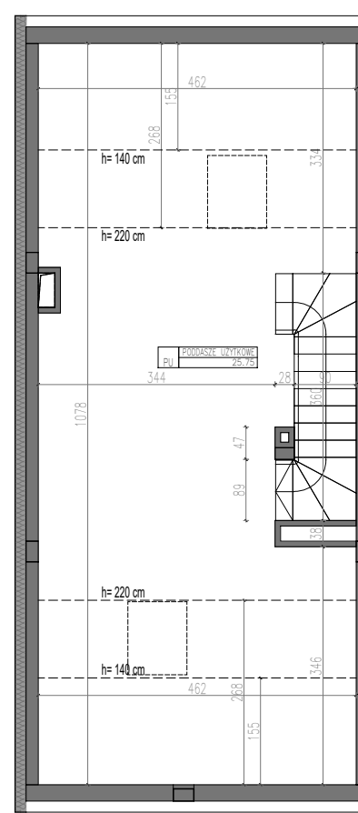
PODDASZE UŻYTKOWE
