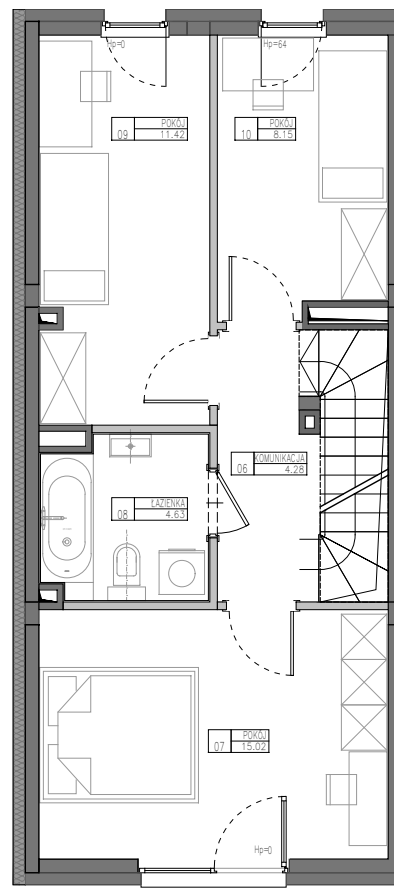
PIĘTRO
