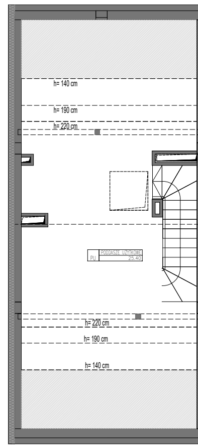
PODDASZE UŻYTKOWE
