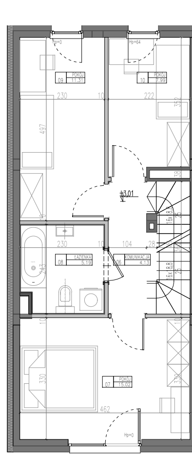
PIĘTRO
