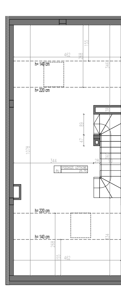
PODDASZE UŻYTKOWE
